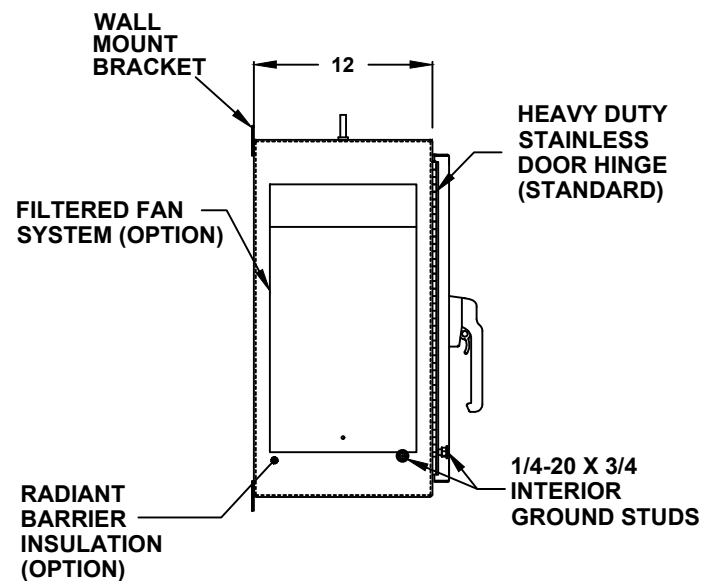
LEFT SIDE
