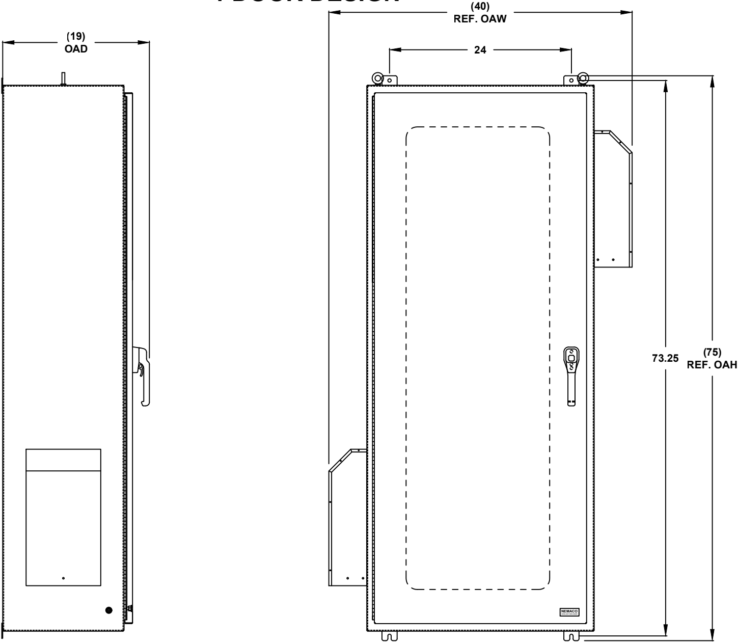
LEFT SIDE
