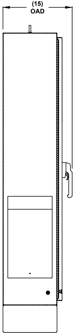
LEFT SIDE
