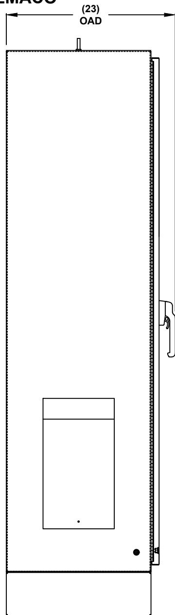
LEFT SIDE
