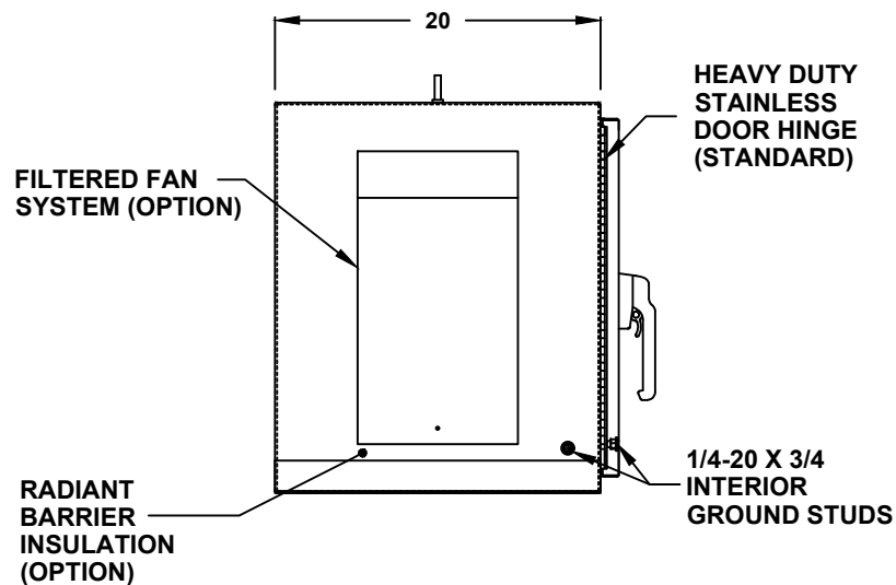
LEFT SIDE
