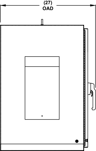
LEFT SIDE
