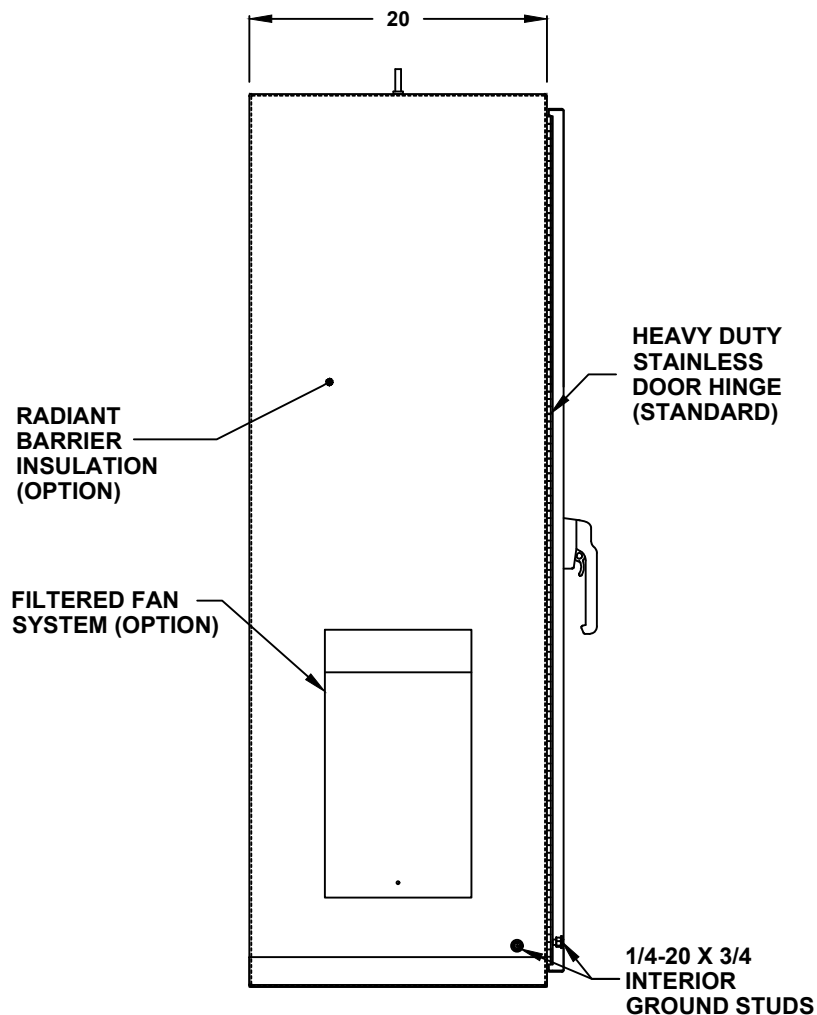
LEFT SIDE
