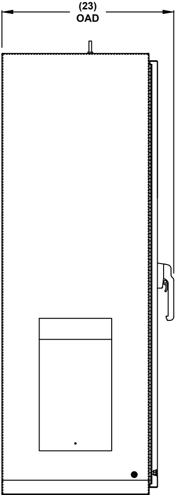
LEFT SIDE
