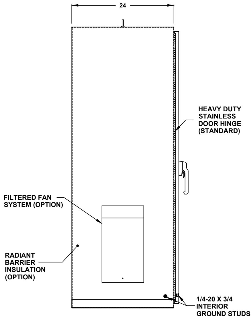
LEFT SIDE
