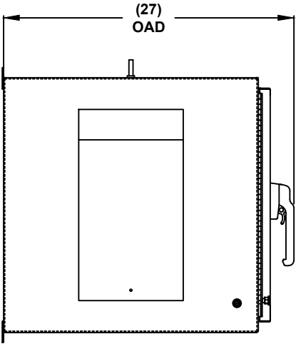
LEFT SIDE
