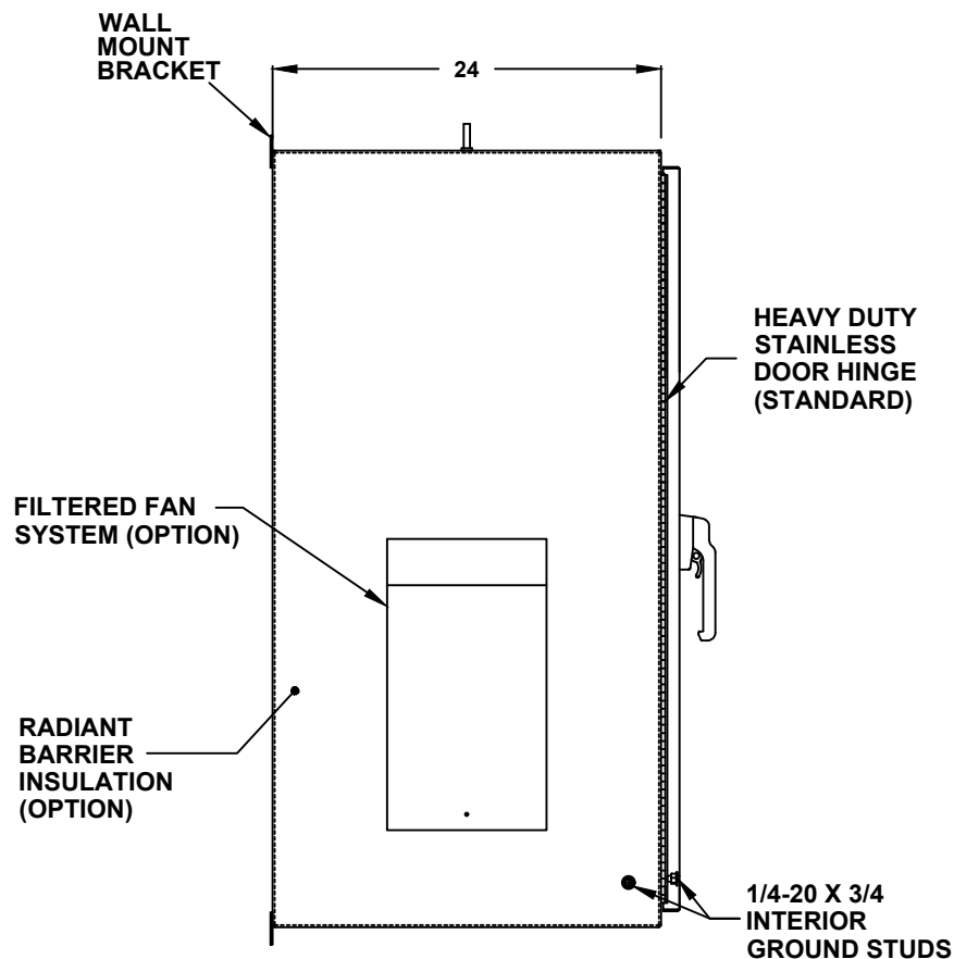
LEFT SIDE
