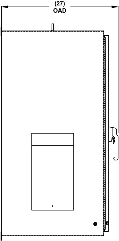
LEFT SIDE
