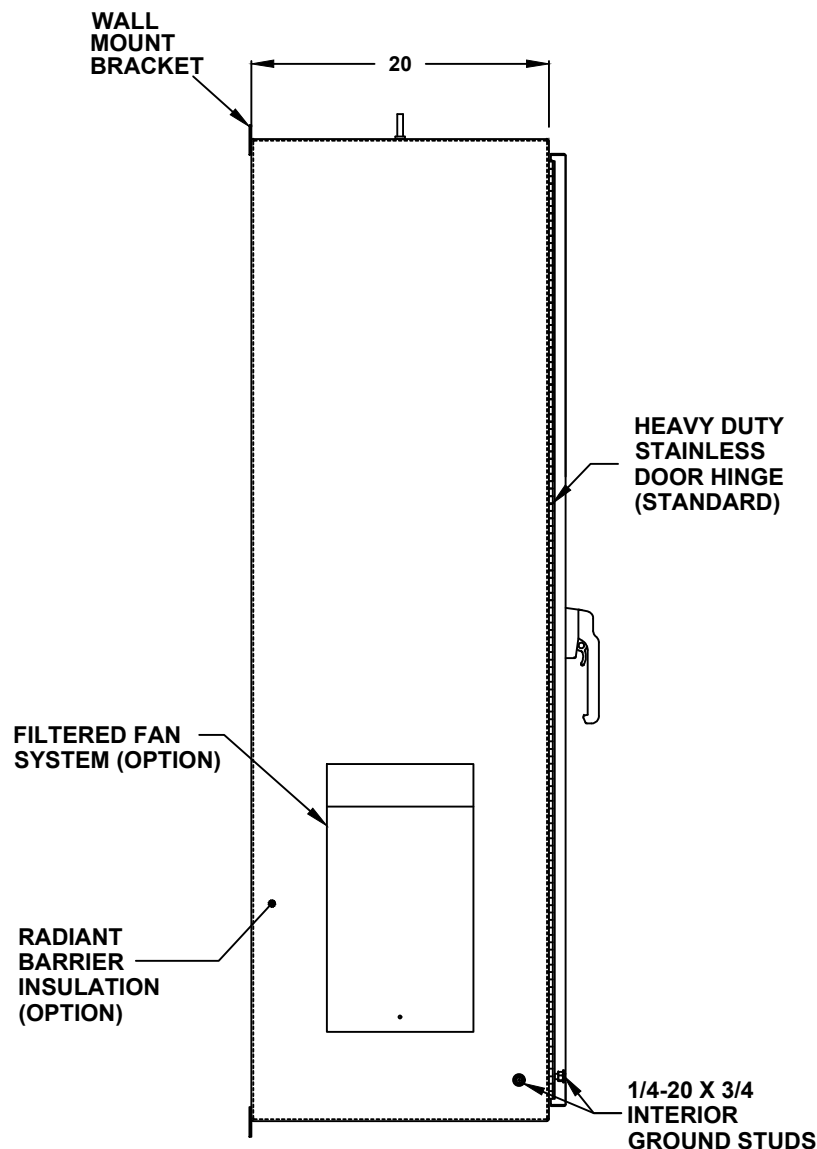
LEFT SIDE
