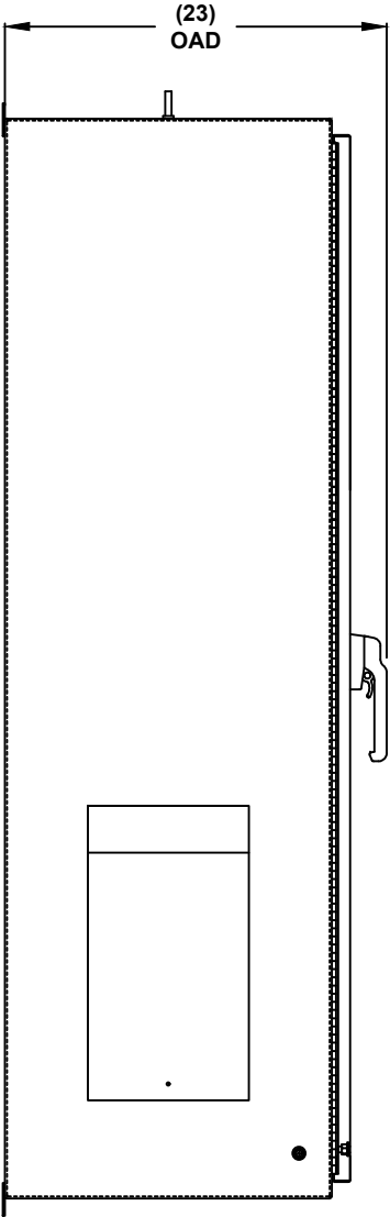
LEFT SIDE
