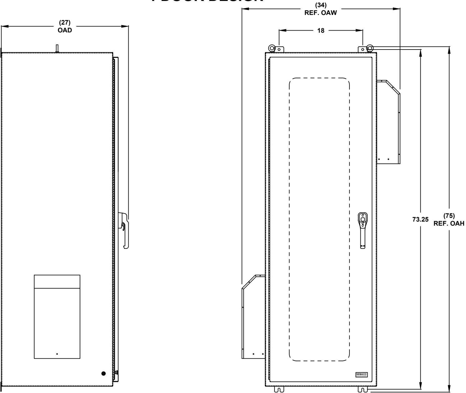
LEFT SIDE
