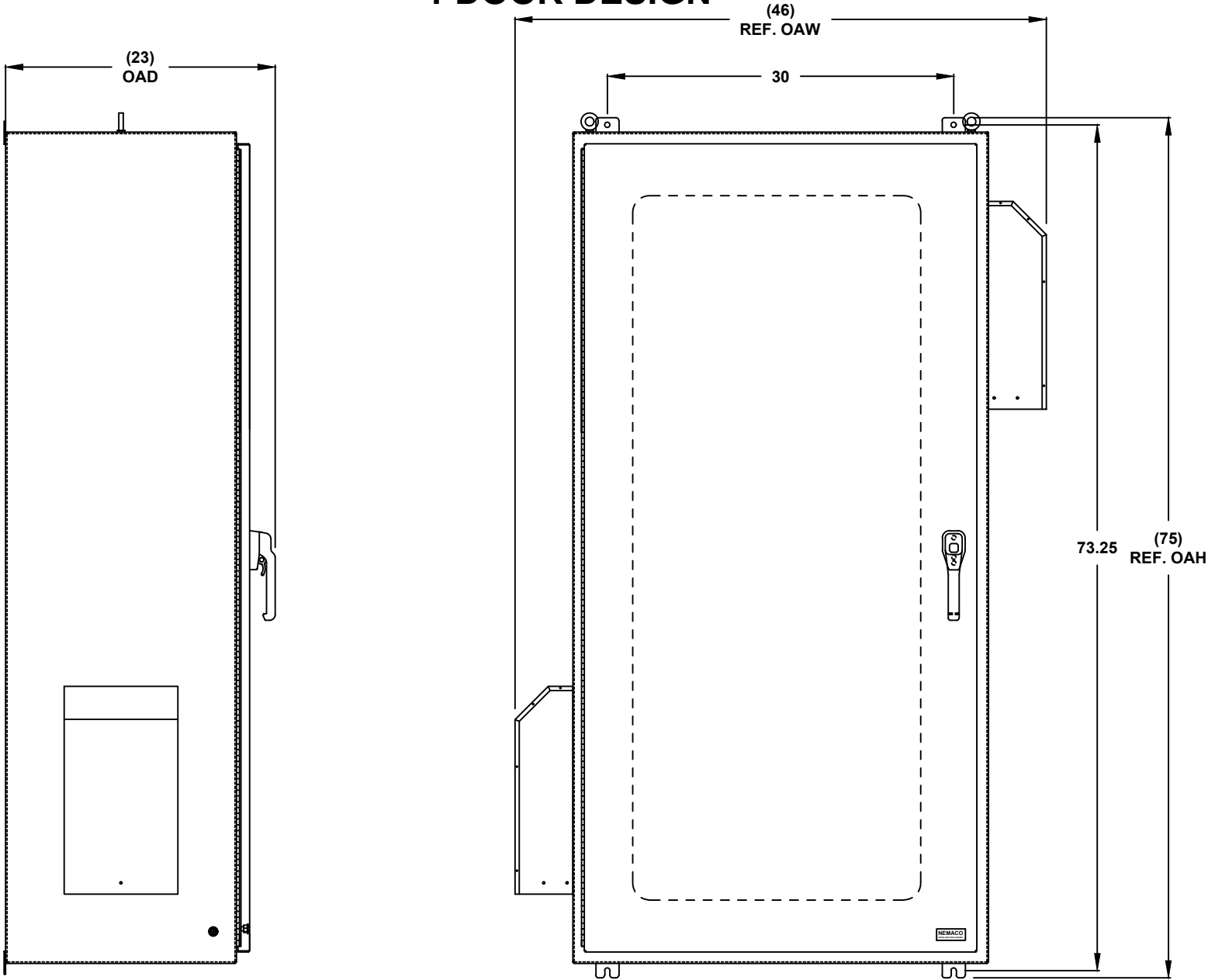
LEFT SIDE
