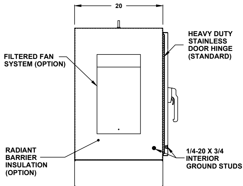
LEFT SIDE
