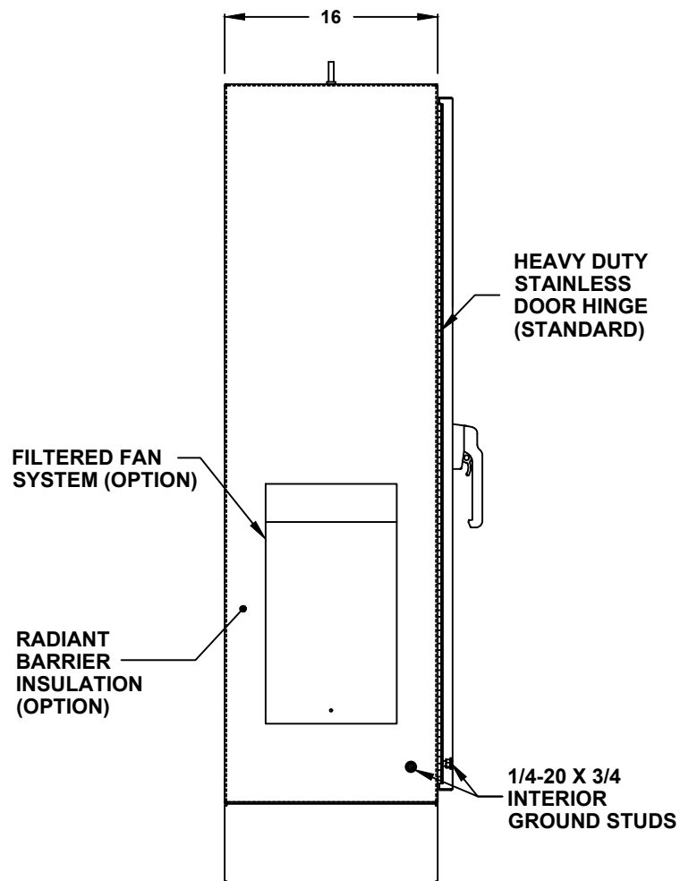
LEFT SIDE
