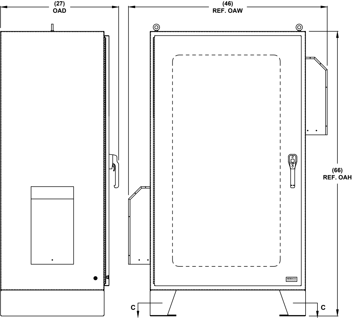
LEFT SIDE
