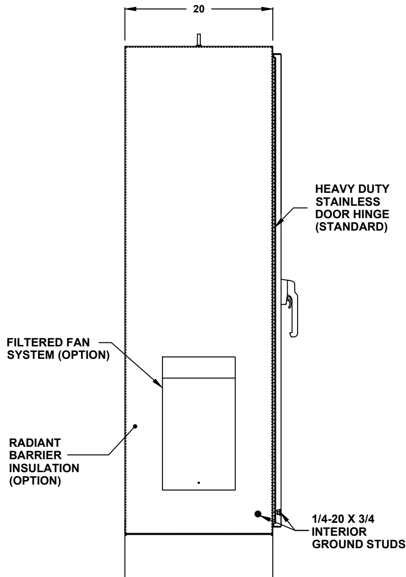
LEFT SIDE
