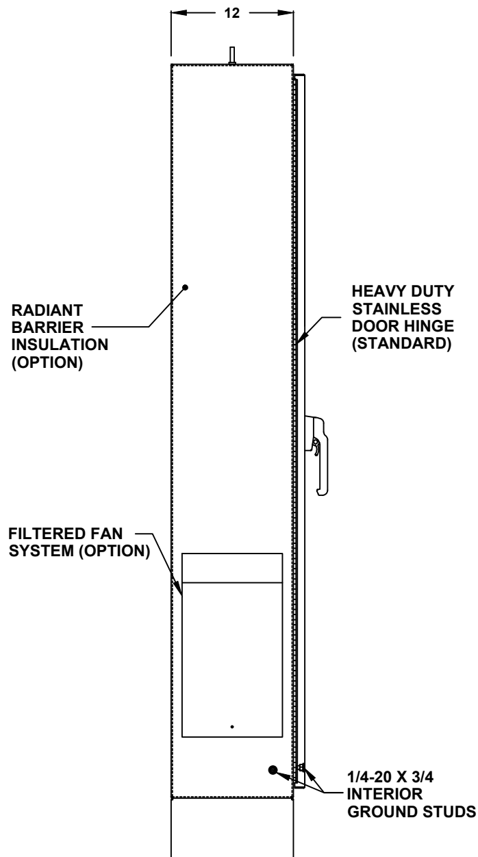
LEFT SIDE
