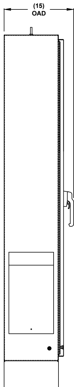
LEFT SIDE
