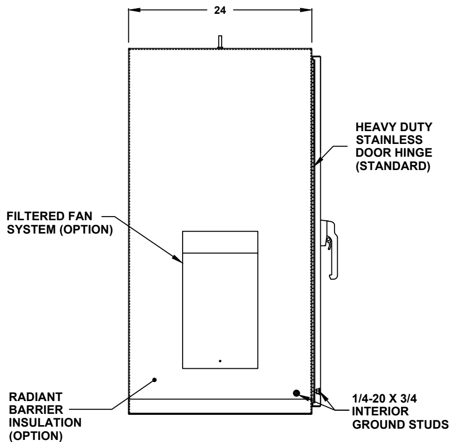
LEFT SIDE
